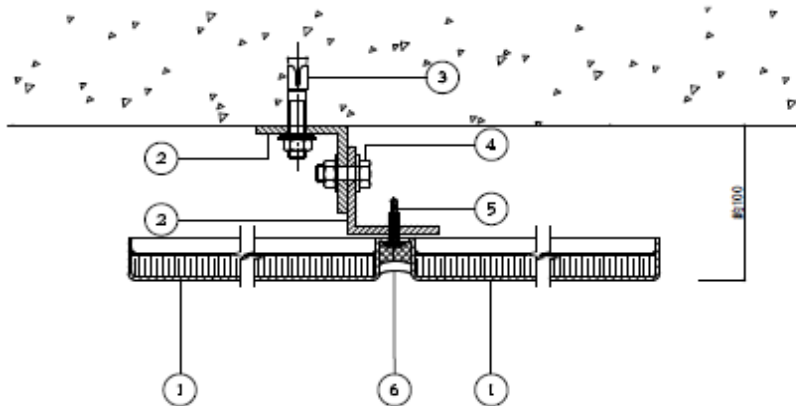
ジョイント断面図
